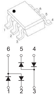
SOT-363
