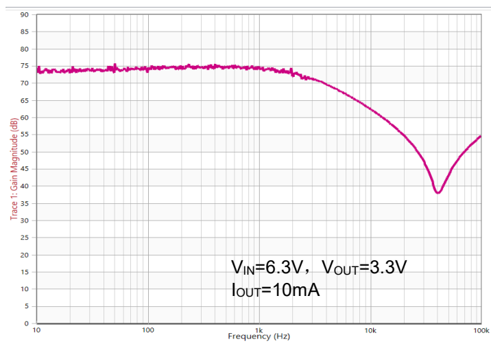
PSRR
