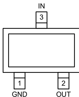
CJ6213-M3N-x.x SOT-23-3L
