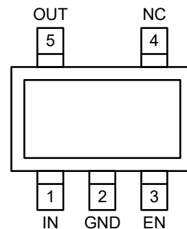
CJ6213-M5N-x.x SOT-23-5L
