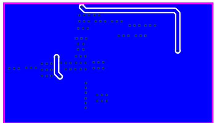
Bottom Layer
