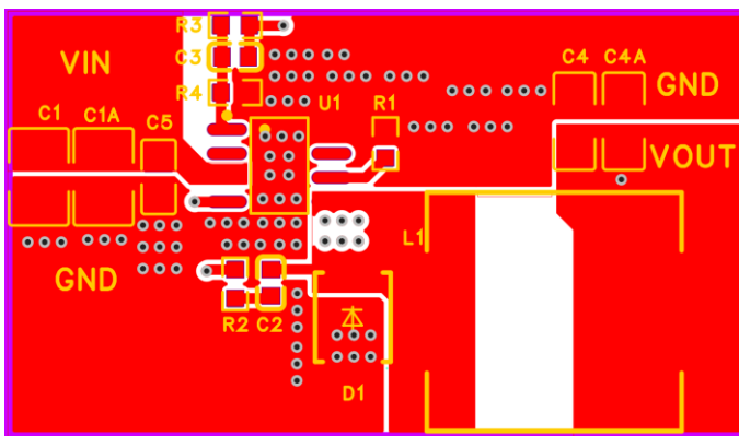
Top Layer
