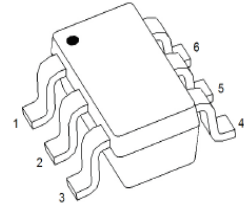
SOT-23-6L
