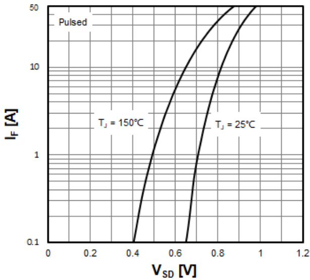
I_s — V_{SD}
