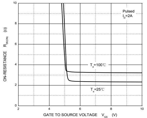
R_{DS(ON)} — V_{GS}
