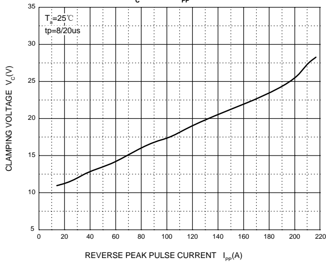
V_C — I_{PP}
