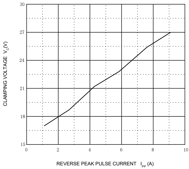
V_c — I_{pp}
